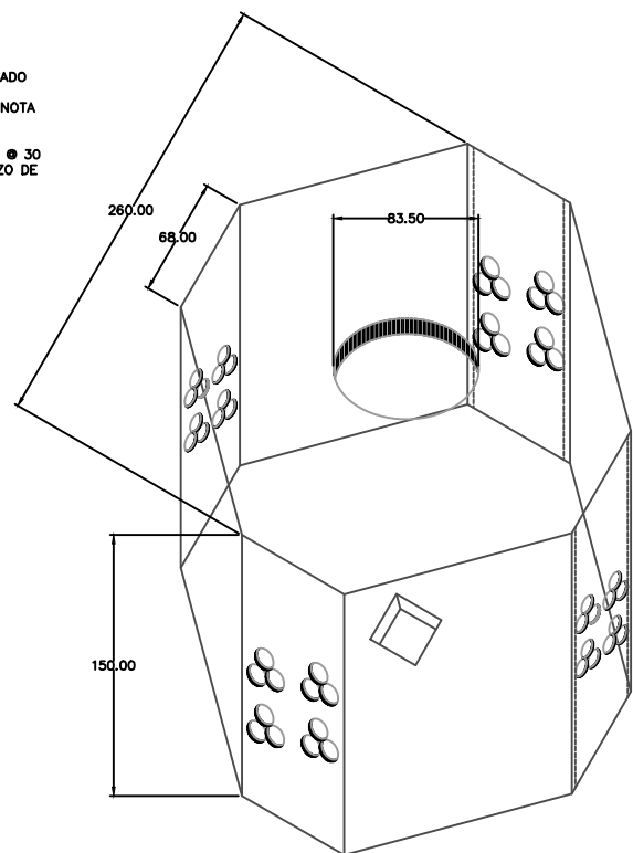
ISOMETRICO
