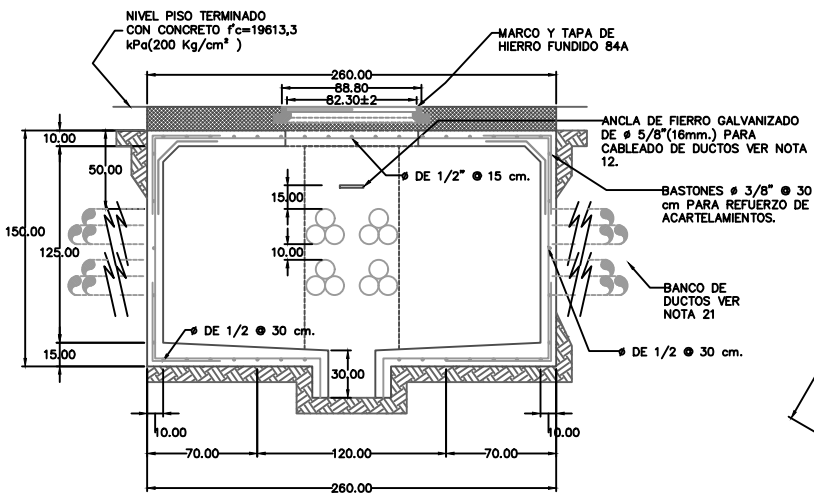
ELEVACIÓN REFUERZO SECCIÓN A-A'
